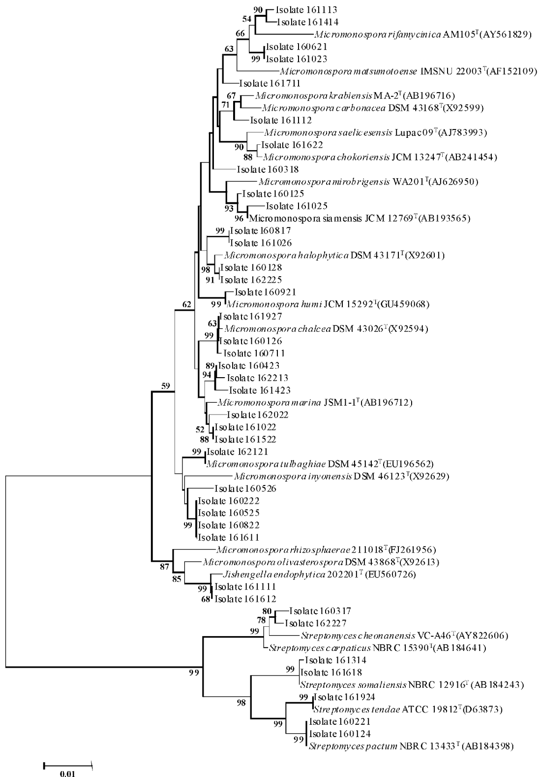
图 1 依据 16S rDNA 序列构建的 42 株代表菌株及其相关菌株的聚类分析图
